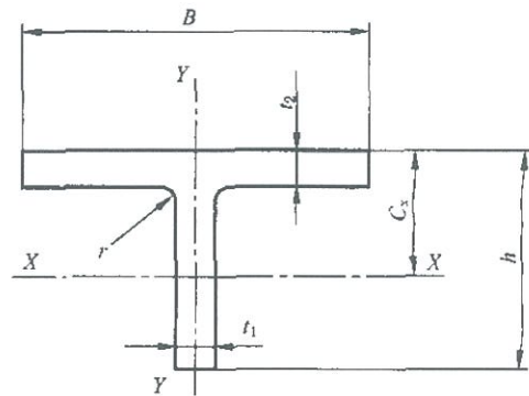
h—高度;B—宽度; t_1 —腹板厚度 t_2 —翼缘厚度; C_x —重心; r —圆角半径
